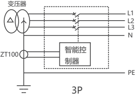
方式四(地电流型)
