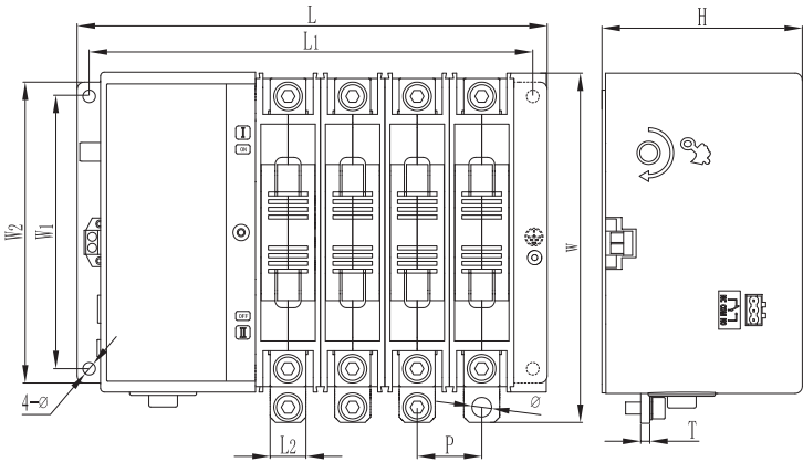
二段式A、B型外形尺寸及安装尺寸
