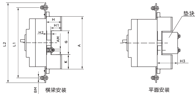
RDHM5-250~800插入式板前断路器外形尺寸
