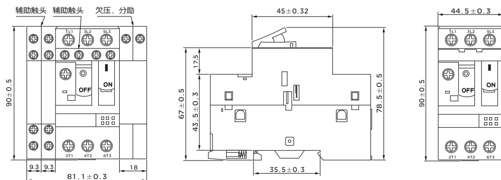
RDS5-32附件及外形尺寸
