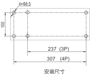
RDW5-1600H安装尺寸
