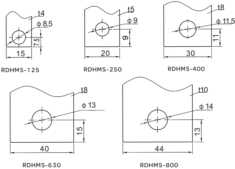
RDHM5系列推荐预制铜排尺寸
