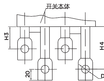
RDHM5-400、630、800板后接线
