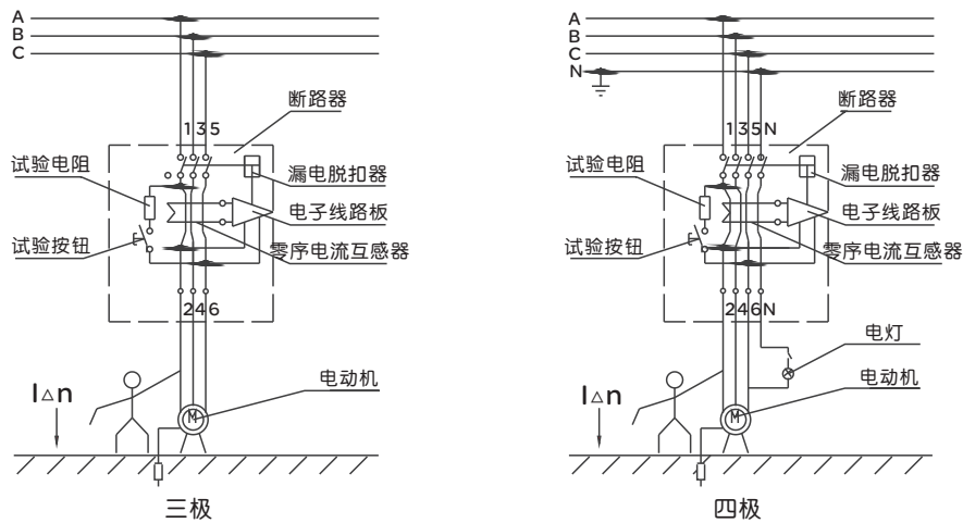
图1 工作原理
