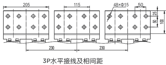
3P水平接线及相间距
