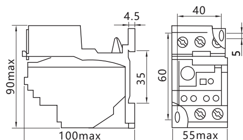
图6 RDR5-38/F外形尺寸图
