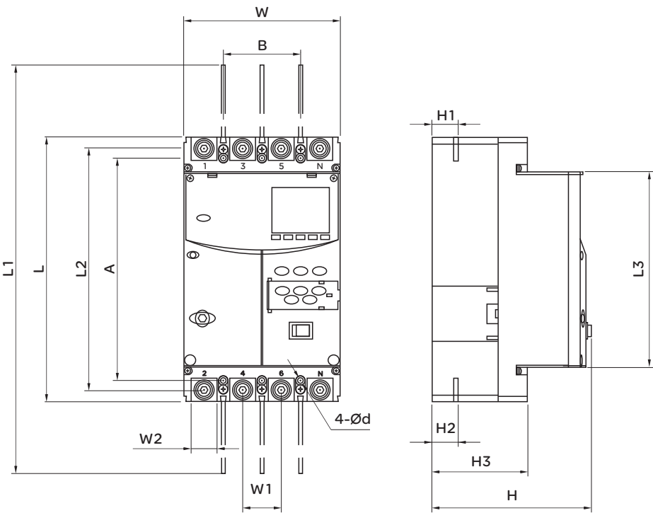
外形及安装尺寸
