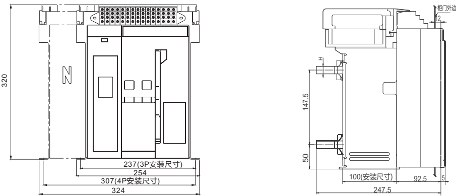
RDW5-1600H安装尺寸
