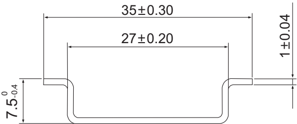
图4 安装轨尺寸
