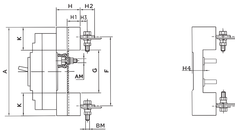
RDM5L-125~800插入式板后断路器外形尺寸
