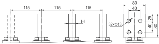
垂直接线及相间距
