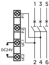
DC24V接线图
