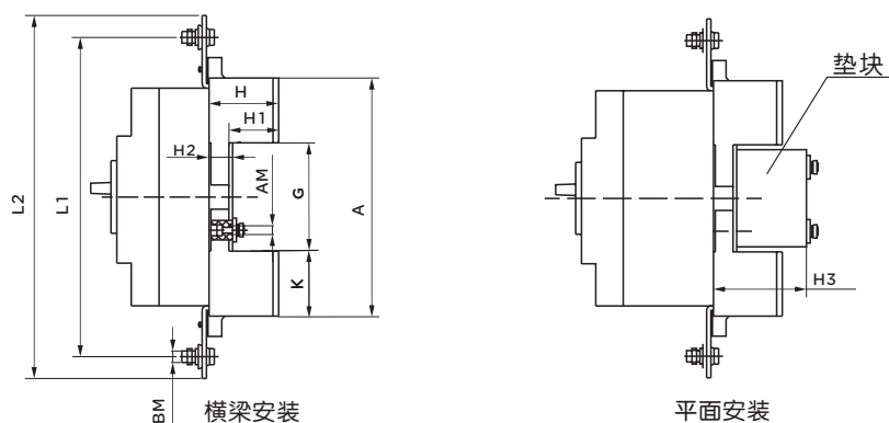
RDM5-125~800插入式板前断路器外形尺寸
