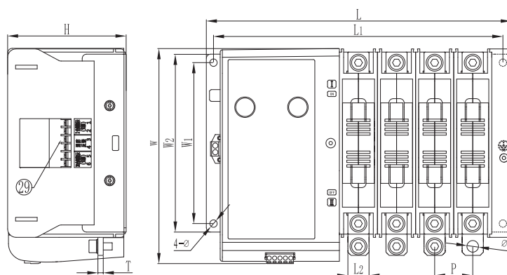
三段式A、B型外形尺寸及安装尺寸
