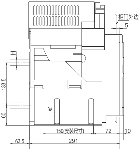
水平接线及外形尺寸
