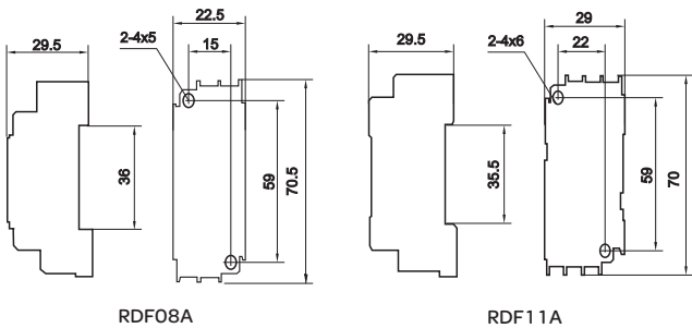
图2:插座外型尺寸、安装尺寸
