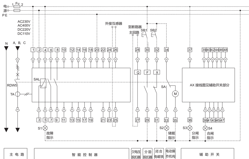
RDW5-1000S/H~1600S、2000-6300S/H系列 M型二次回路接线图
