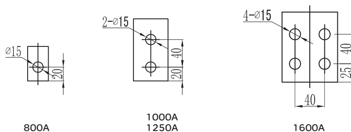
铜排连接开孔尺寸
