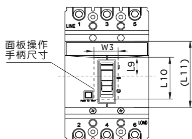
RDHM5系列板后接线外形及安装尺寸
