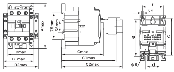
图6 RDC5-40 ~ 95
