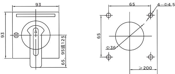
方形延伸旋转手柄开孔尺寸图
