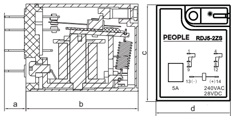
图1:继电器外型尺寸
