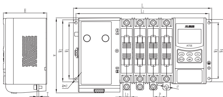
二段式C型外形尺寸及安装尺寸
