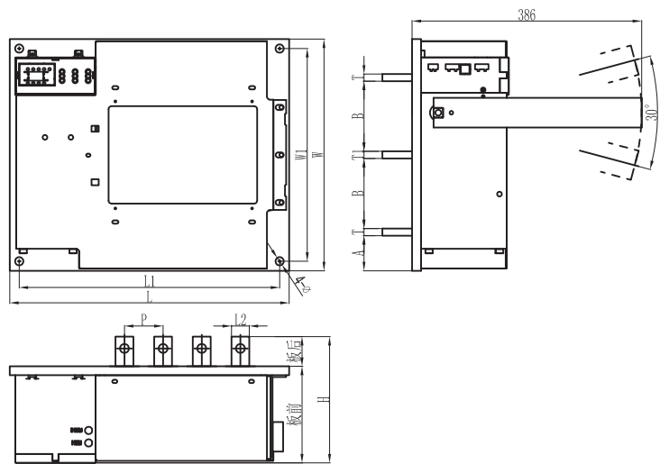
二段式、三段式A、B、C型外形安装尺寸
