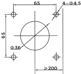
方形延伸旋转手柄开孔尺寸图
