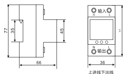
2P液晶型外形及安装尺寸
