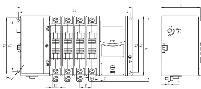
三段式C型外形尺寸及安装尺寸
