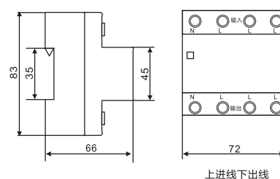
3P+N外形及安装尺寸
