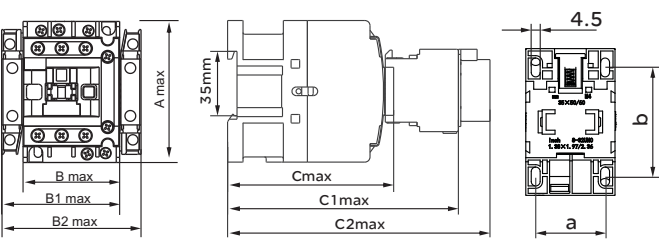
图5 RDC5-06 ~ 38
