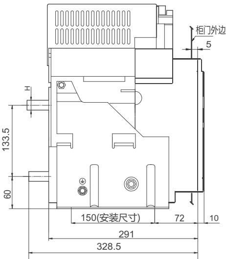
水平接线及外形尺寸
