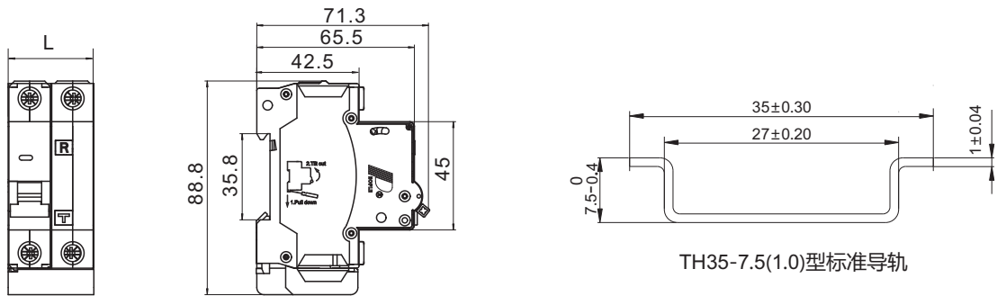
外形及安装尺寸
