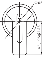
圆形延伸旋转手柄开孔尺寸图
