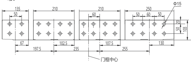
4P水平接线及相间距
