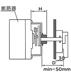
图5 手动操作机构尺寸图
