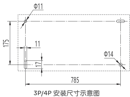
3P/4P 安装尺寸示意图
