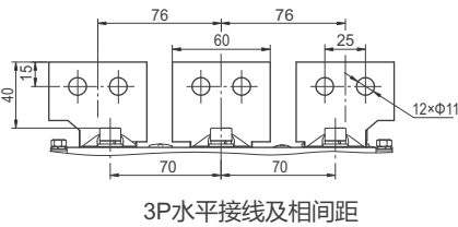
RDW5-1600H安装尺寸
