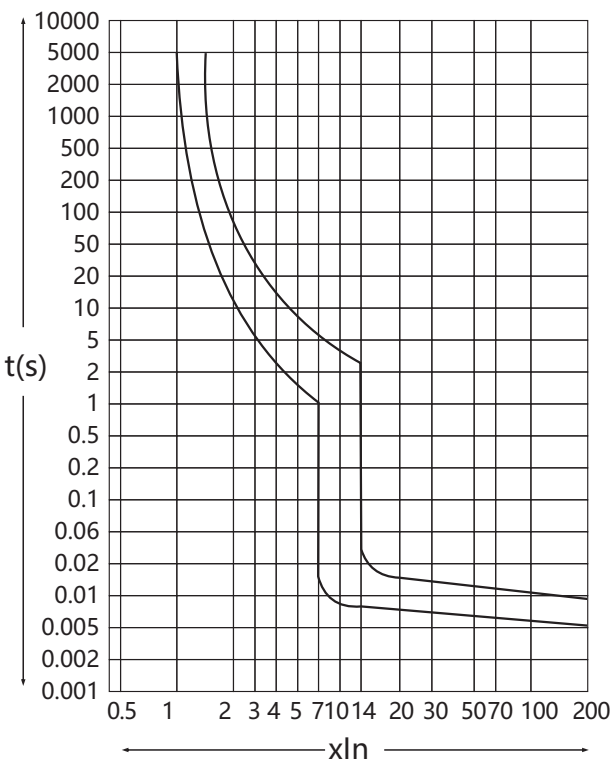
图2 时间电流特性曲线
