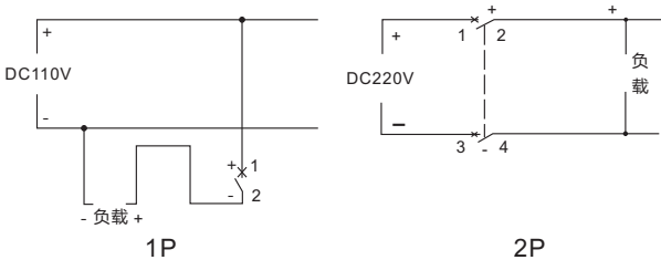
图2 接线方式
