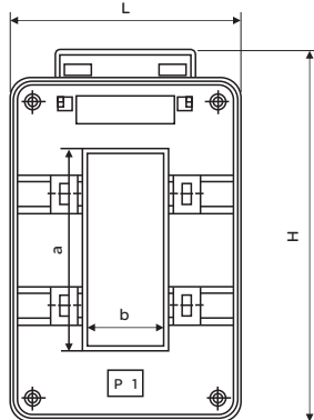
图2 LMK5-O.66 (60~130型)
