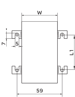
图1 LMK5-O.66 (30~50型)
