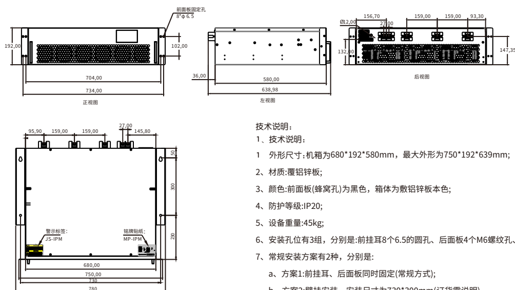
RD-PQC-SVG/150kvar-0.4/4L-N外形尺寸图
