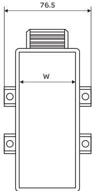
图2 LMK5-O.66 (60~130型)
