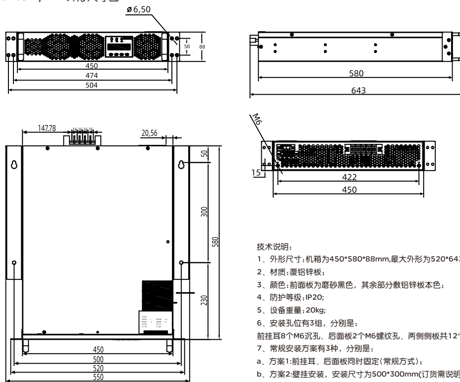
RD-PQC-SVG/30kvar-0.4L/4L-N外形尺寸图
