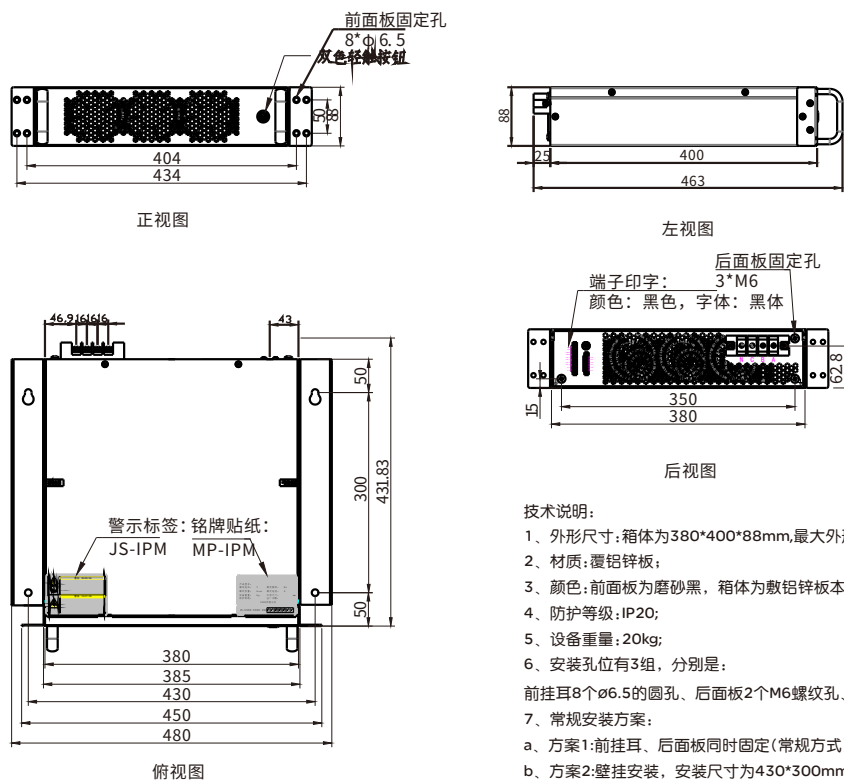
RD-PQC-SVG/30kvar-0.4/4L-S外形尺寸图
