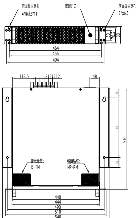
RD-PQC-APF/75A-0.4/4L-S外形尺寸图
