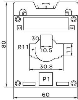
图2：30型正视
