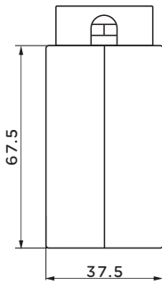
图3：侧视
