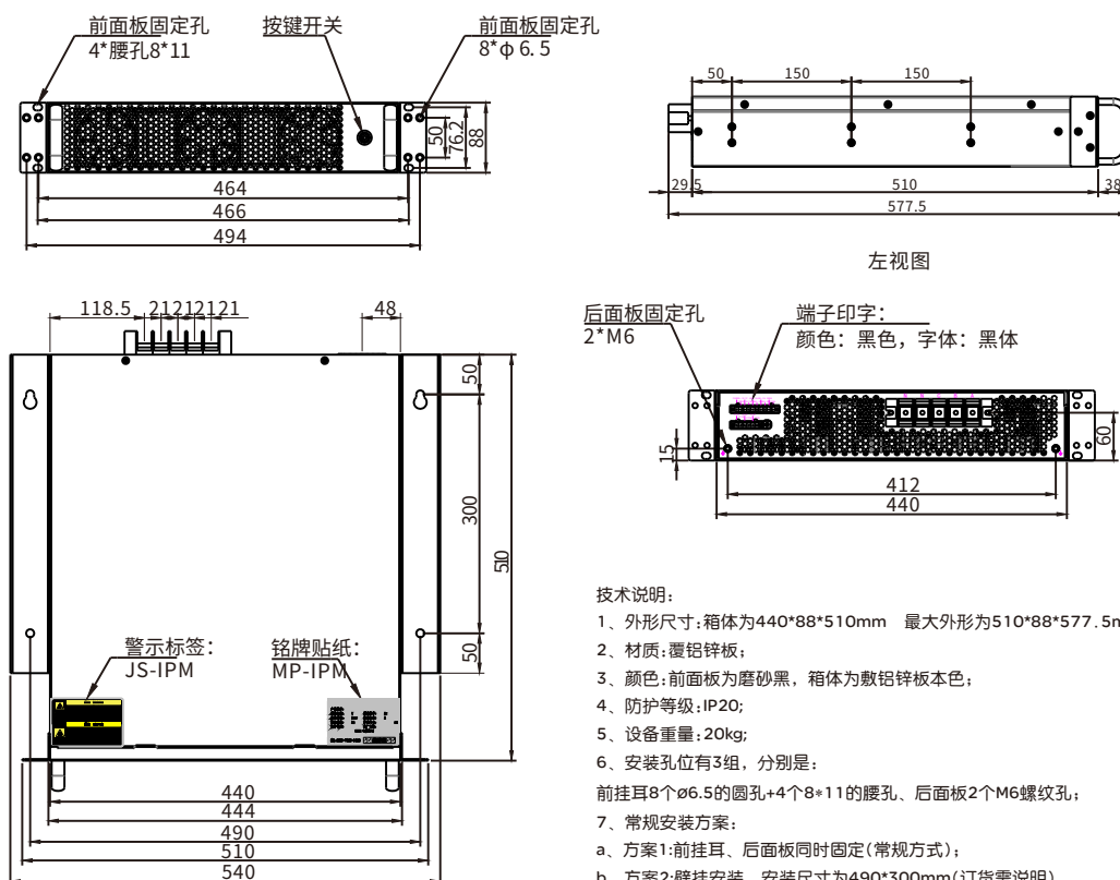
RD-PQC-SVG/50kvar-0.4/4L-S外形尺寸图
