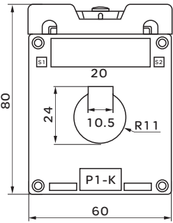
图1：20型正视
