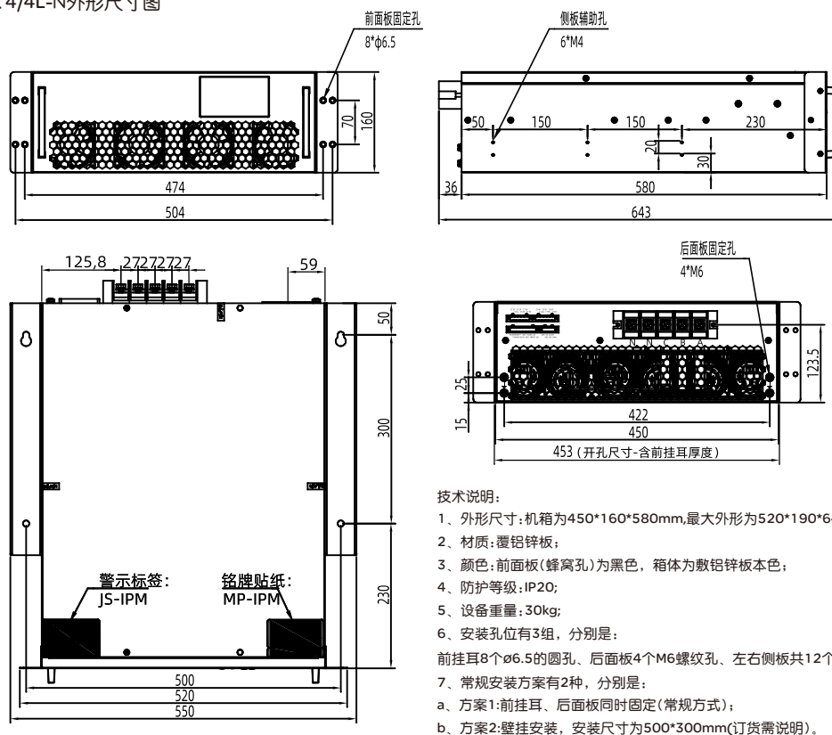
RD-PQC-APF/100A-0.4/4L-N外形尺寸图
