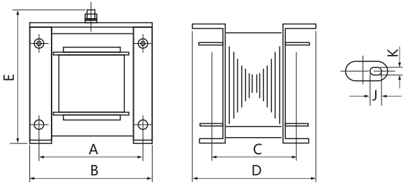
图4 JBK4系列产品的外形及安装尺寸（见表3）
