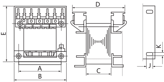
图3 JBK3系列产品的外形及安装尺寸（见表2）
