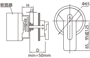
图6 手动操作机构安装尺寸图
