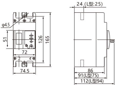
图8b RDM1L-250M/2300
