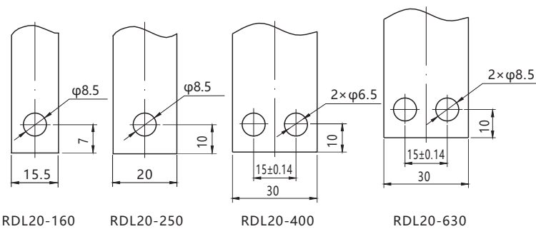
图2 预制铜排开孔尺寸
