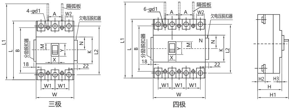
图7 RDM1-80~800板前接线外形及安装尺寸
