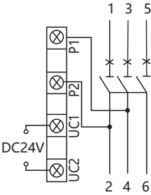
图1 DC24V接线图
