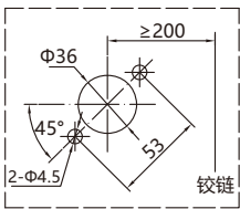
圆形延伸旋转手柄 开孔尺寸图
