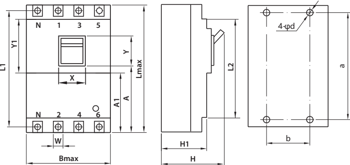
图1 RDL20漏电断路器的外形及安装尺寸
