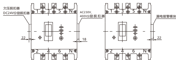
图9 附件装置尺寸 注：欠压脱扣器、分励脱扣器安装位置具体见表2,漏电报警模块固定安装在右侧。
