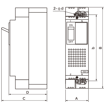
图2 二极断路器外形尺寸和安装尺寸
