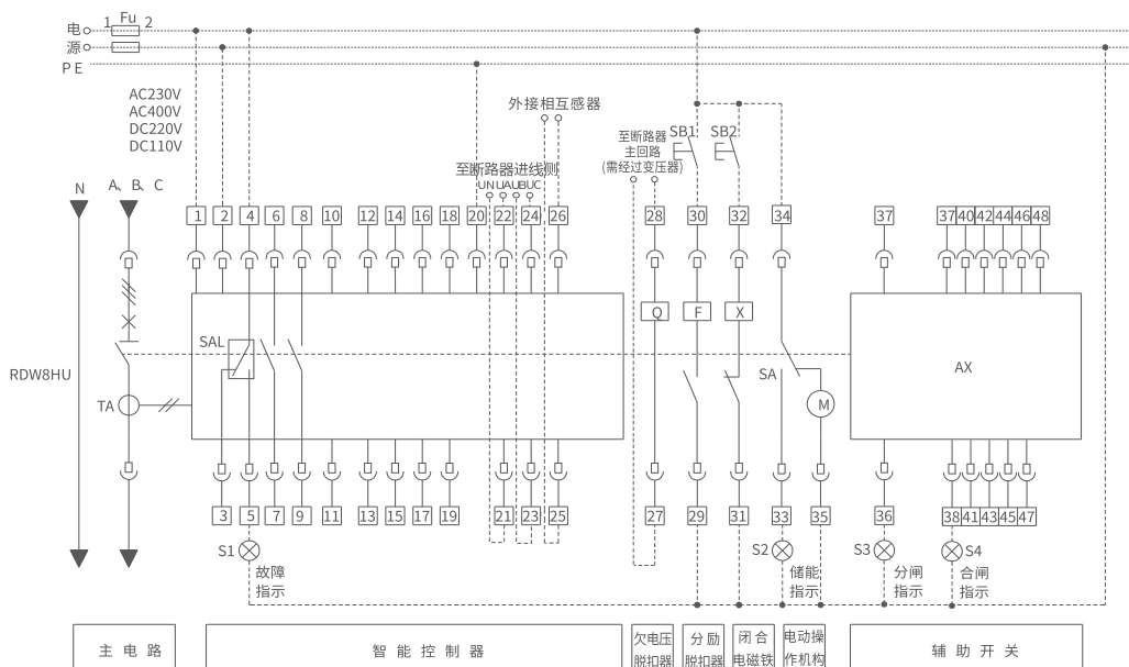
RDW8HU-2500/4000/6300 R型二次回路接线图
