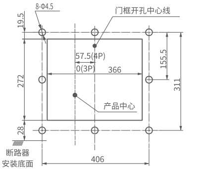
RDW8DC-4000固定式断路器面板开孔尺寸
