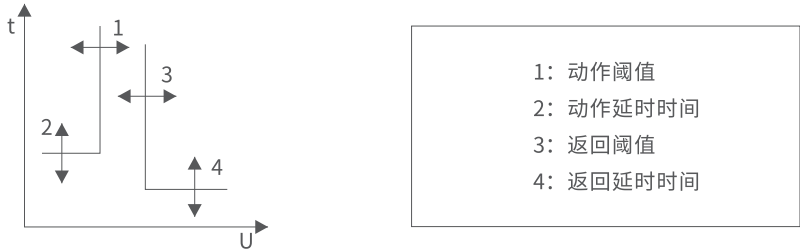
图1 欠压保护动作原则
