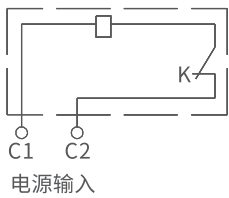
图1 AC230V、400V、DC24V接线图
