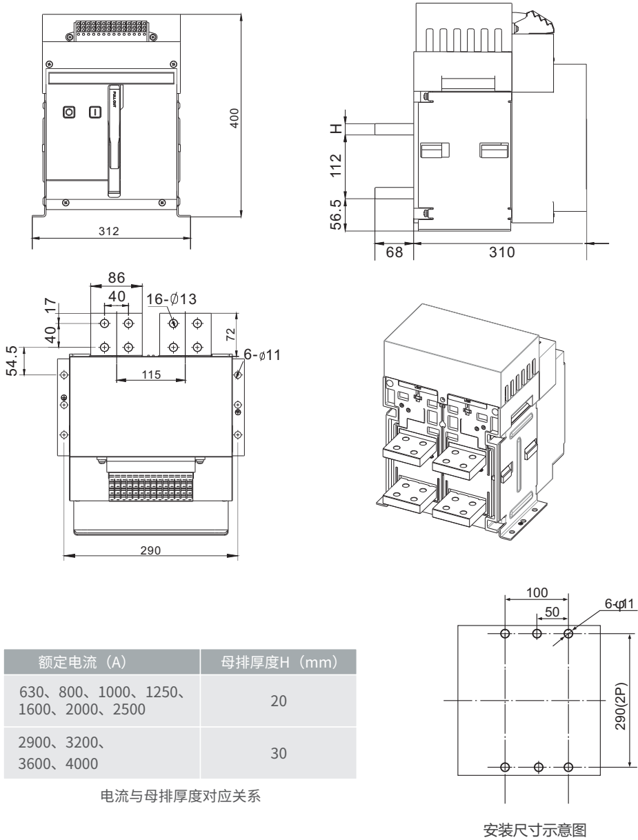
RDW8GDC-4000框架隔离开关（固定式）
