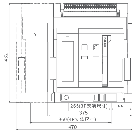
RDW8DC-2500智能型万能式断路器（抽屉式）
