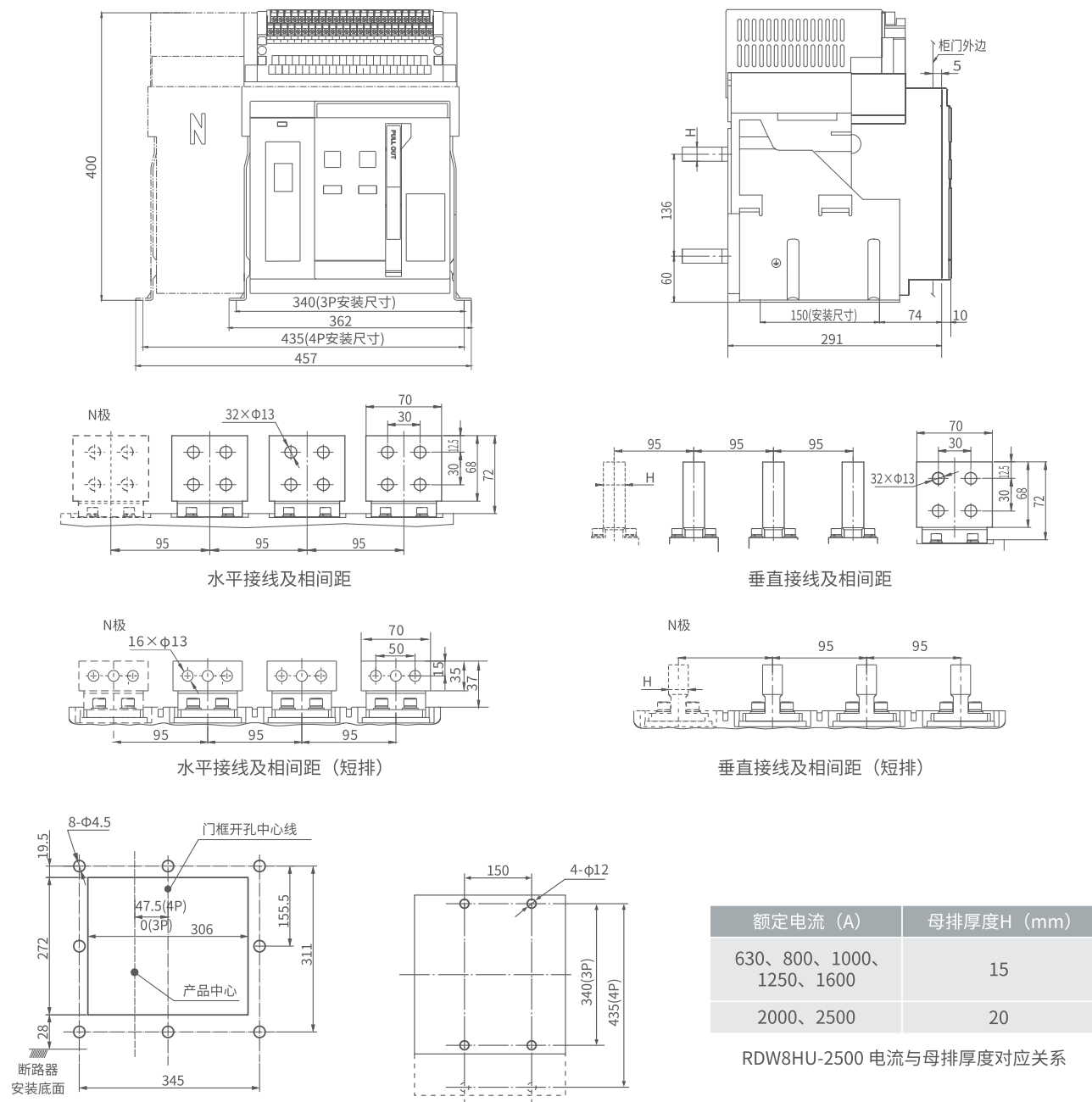
RDW8DC-2500固定式断路器面板开孔尺寸
