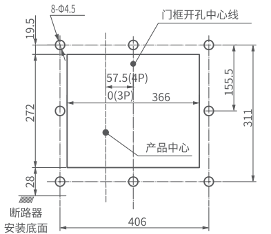
RDW8HU-4000固定式断路器面板开孔尺寸
