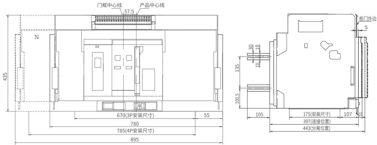
RDW8HU-6300智能型万能式断路器（抽屉式）
