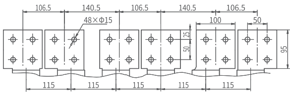
3P水平接线及相间距
