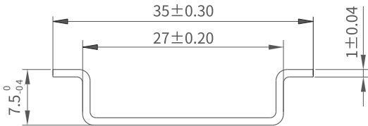
图 3 安装轨尺寸
