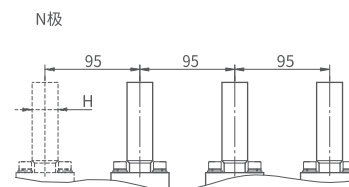
垂直接线及相间距
