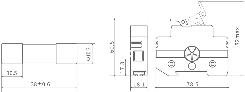
图1 熔断体
