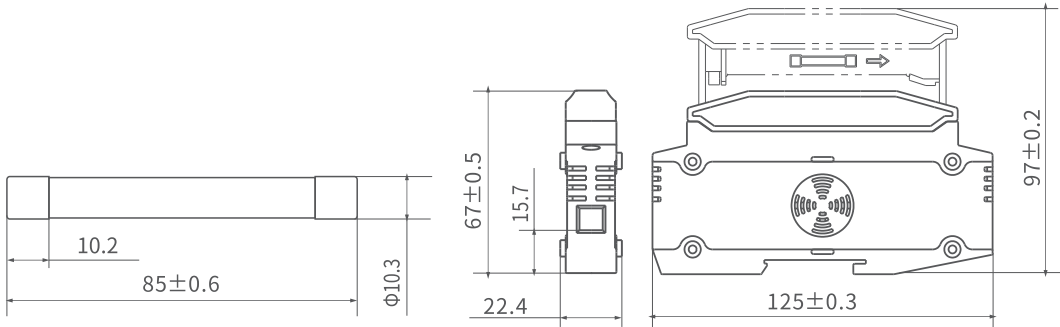
图3 熔断体
