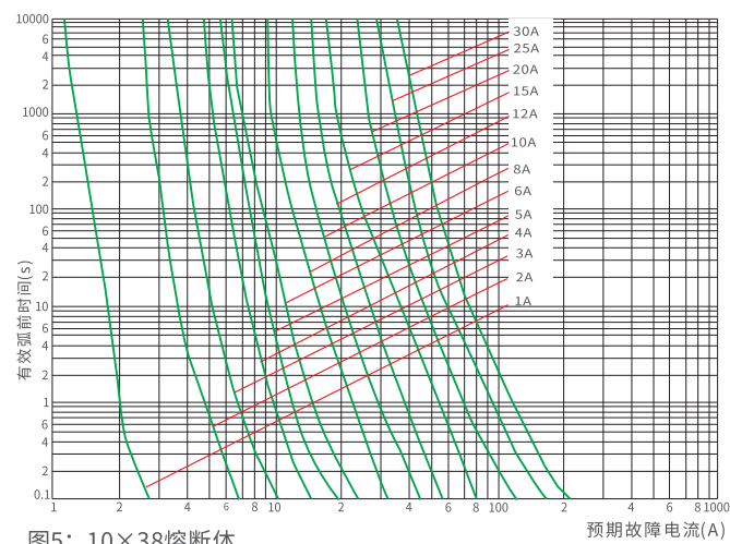
图5：10×38熔断体
