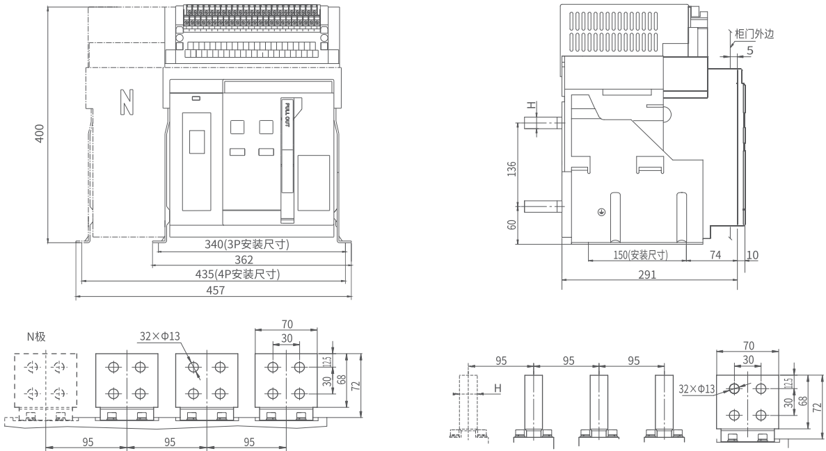
水平接线及相间距
