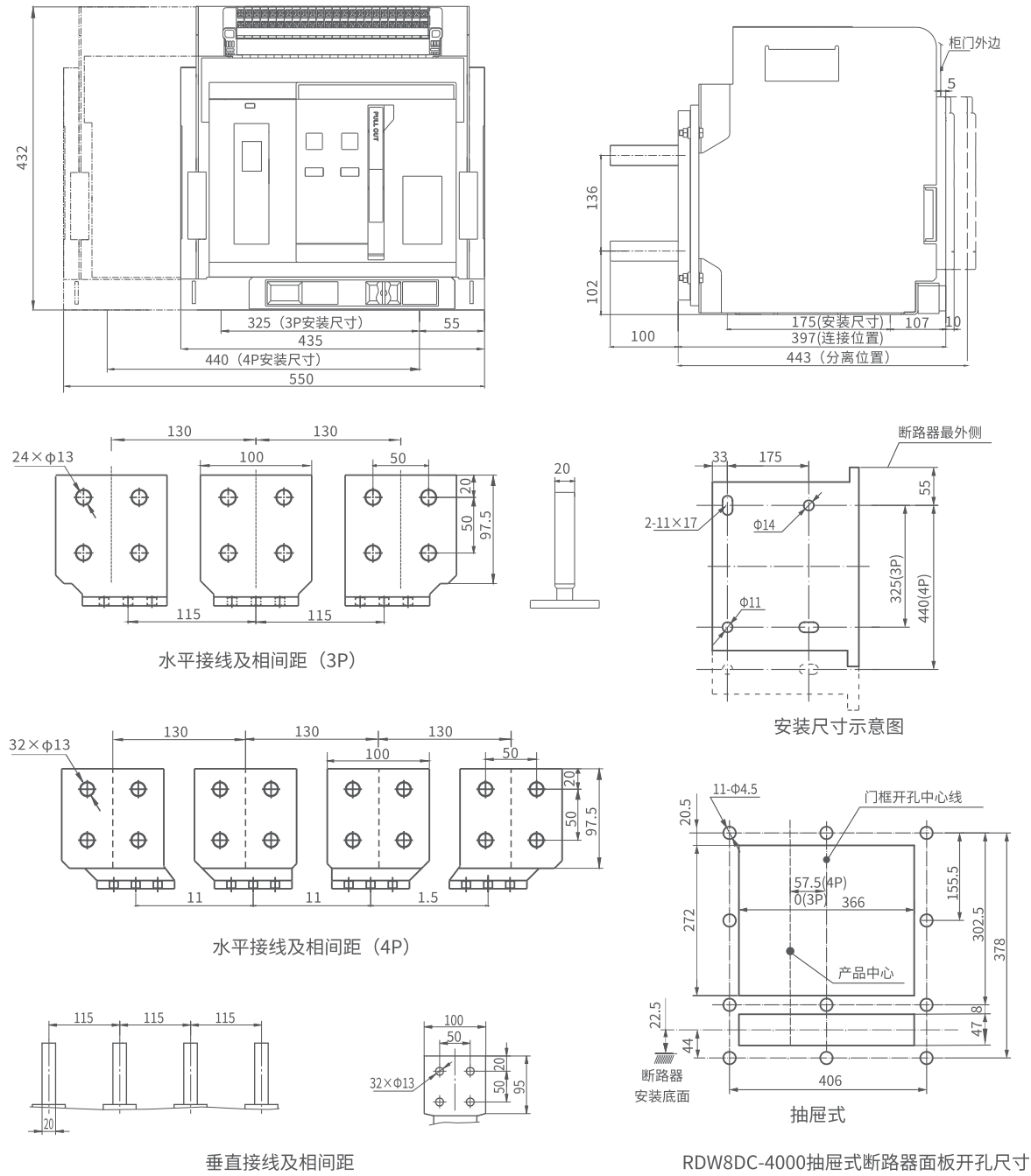
RDW8DC-4000抽屉式断路器面板开孔尺寸
