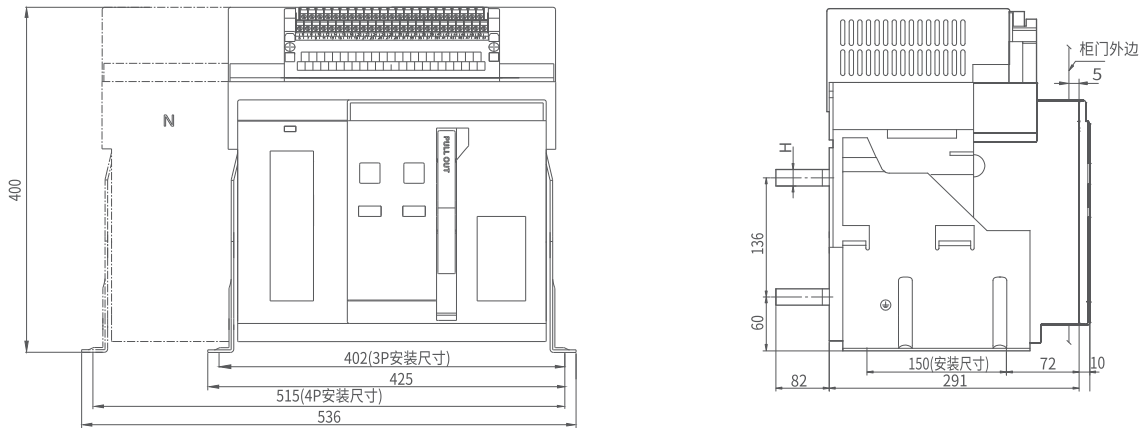
RDW8HU-4000智能型万能式断路器（固定式）
