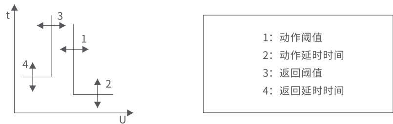
图2 过压保护动作原则
