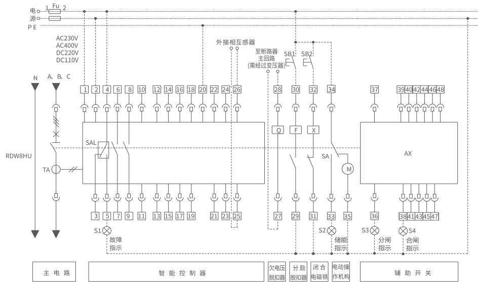
RDW8HU-2500/4000/6300 M型二次回路接线图
