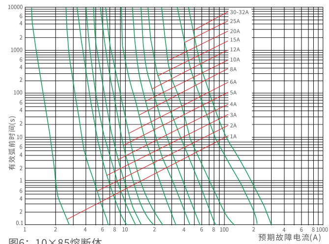
图6：10×85熔断体
