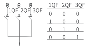
方式四：三路电源一路负载联锁 电路图 可能的运行方式
