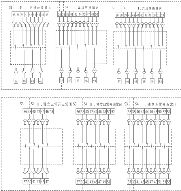
RDW8HU-2500/4000/6300 M型二次回路接线图端子功能与符号释义
