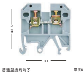
普通型接线端子 厚度6
