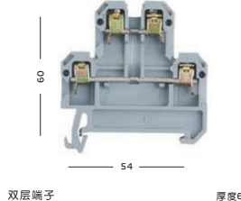
双层端子 厚度6
