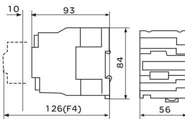
图3 CJX2s-25
