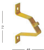
安装轨托架 厚度18
