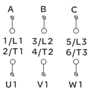
控制三相电动机接线图
