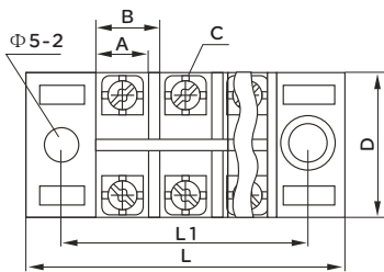
JH(TB)-4503
