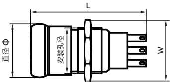
焊接式
