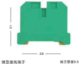
微型接线端子 端子厚度9.5
