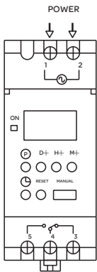
线路图
