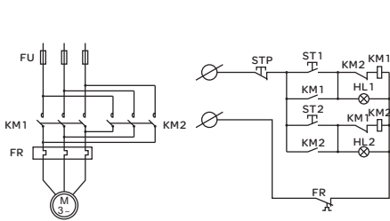
图1 RDQ12/NH可逆电磁起动器电气原理图
