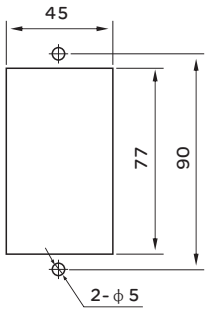
图5 JS14A-□/M系列 面板式安装尺寸
