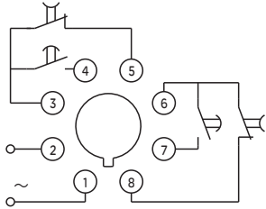
图2 JS14S-C (JS14C、JS14CL) 接线图
