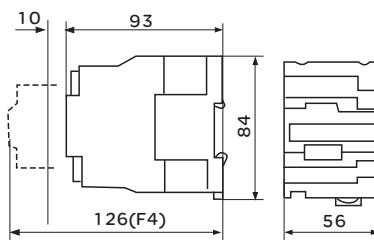
图3 CJX2-25
