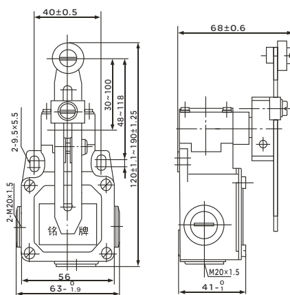
图18 L XK3-20H/T
