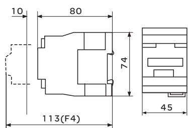
图1 CJX2-09、12
