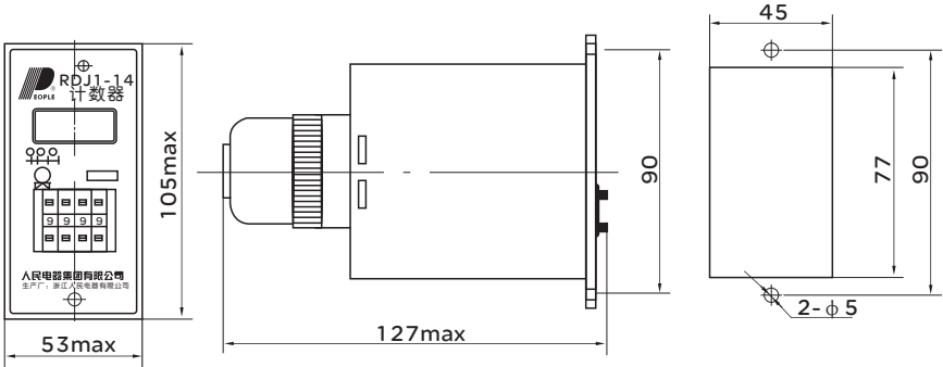
图4 RDJ1-14外形及安装尺寸
