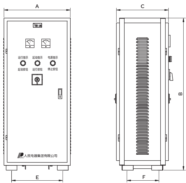
图4 90kW~300kW
