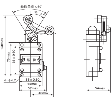
图6 LX19-232
