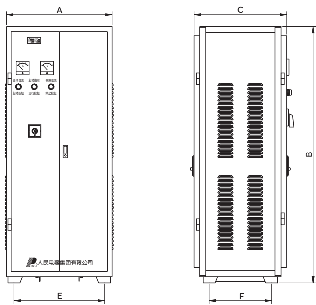
图4 90kW~300kW
