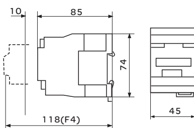
图2 CJX2s-18
