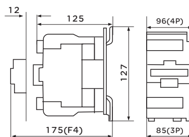
图6 CJX2s-80、95
