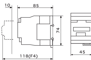
图2 CJX2-18
