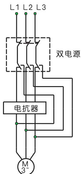
图1: 接线原理图
