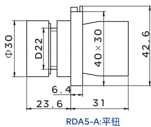
RDA5-A:平钮
