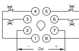
工作电源
