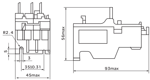
图4 JRS1-25/Z热过载继电器外形及安装尺寸
