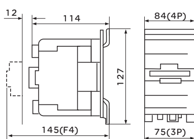
图5 CJX2s-40、50、65
