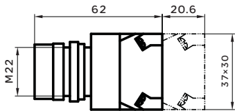
RDA37高头钮
