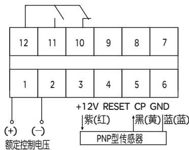
图1 RDJ1-9 接线图
