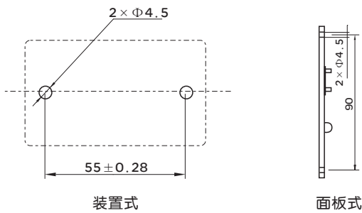
图3 安装尺寸图
