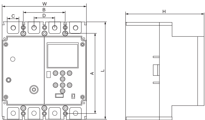
短款尺寸图
