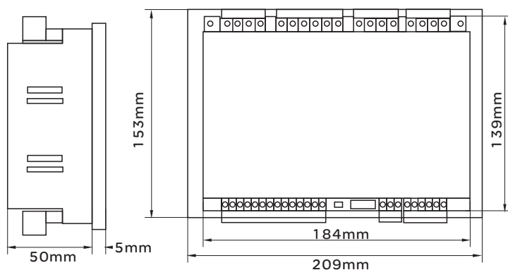
控制器外形尺寸
