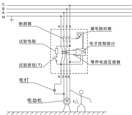
图1 工作原理图
