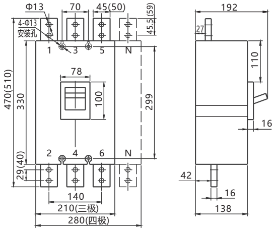
图11 RDM1-1250/1600断路器外形尺寸及安装尺寸 (括号内为1600尺寸)
