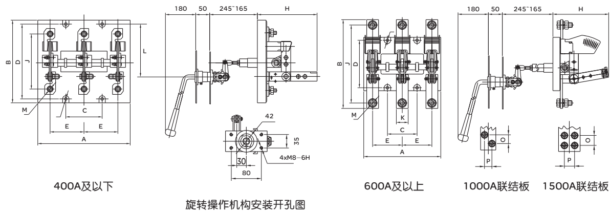
HD13-/BX中央旋转操作机构刀开关外形及安装尺寸见图10、表11
