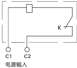
图2 AC230V、AC400V,50Hz接线图
