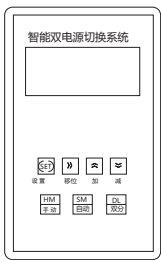
分体式控制器开孔尺寸:87X147; 控制器线长1.8米。
