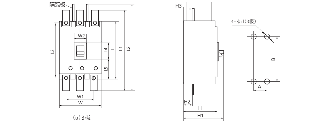
图1a 板前接线外形及安装尺寸
