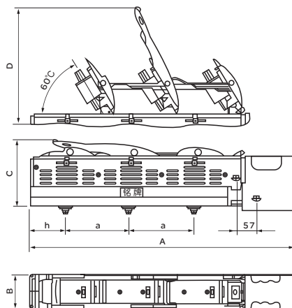
图2 RDHG2B-250、400、600/32(三相同时分断)
