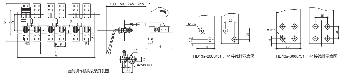
HD13s BX中央旋转操作机构刀开关外形及安装尺寸见图4、表4
