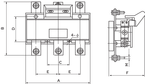
图1 HD11F-200~1500/3
