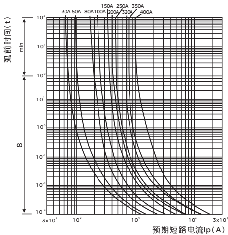
RS0、RS3系列熔断体时间-电流特性曲线
