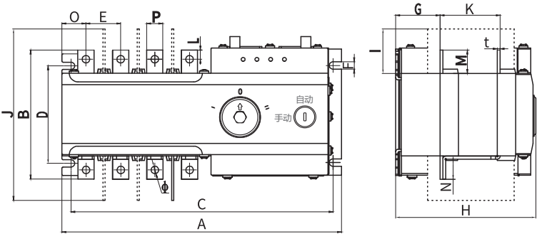
RDH5DS-125外形
