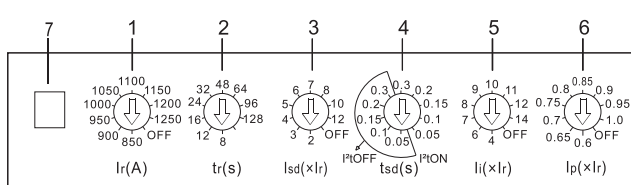
RDM1E-1250, I_n=1250A 电子式脱扣器
