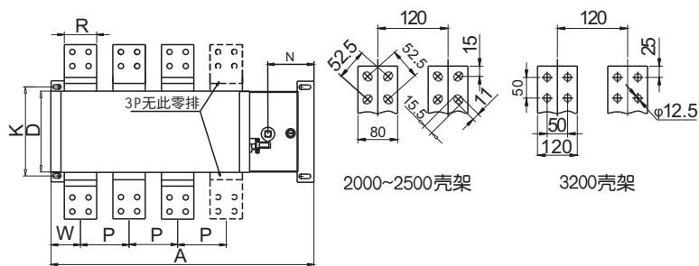
RDH5D-2000-3200外形及尺寸
