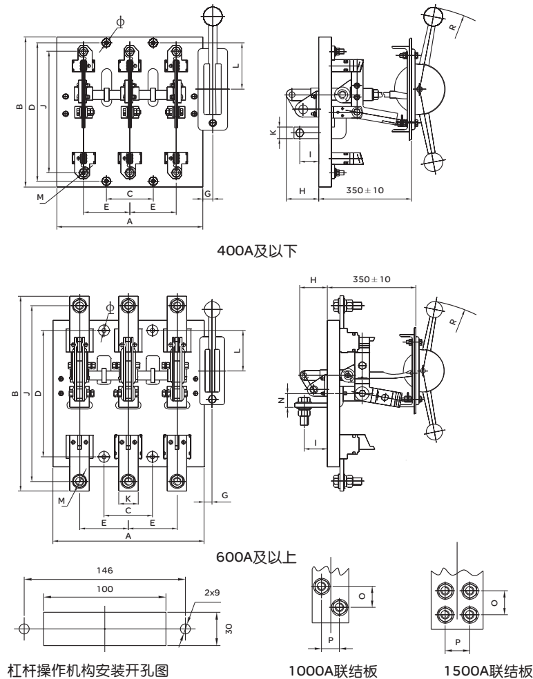
HS12侧方正面杠杆操作机构刀开关外形及安装尺寸见图6、表7
