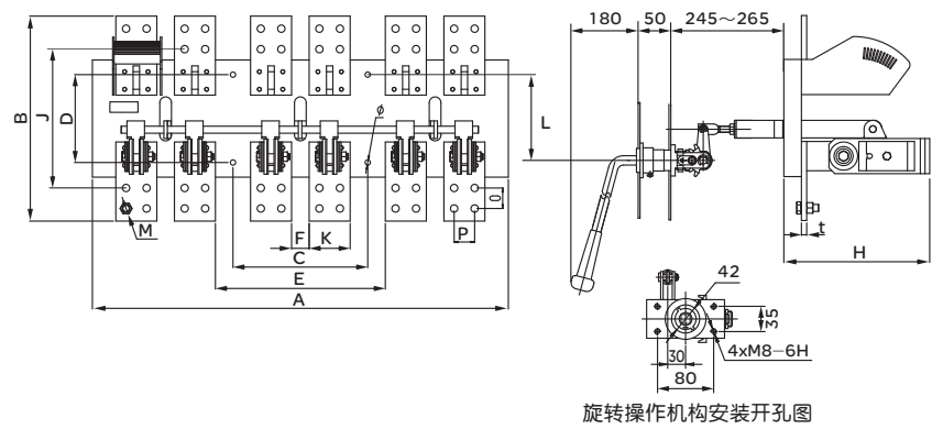
HD13-/BX中央旋转操作机构刀开关外形及安装尺寸见图11、表12
