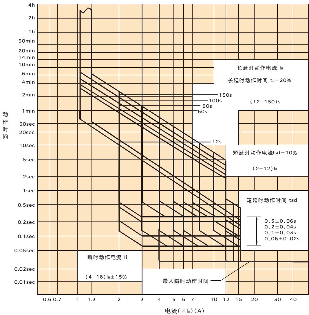
图1 RDM1E-125-1250型脱扣特性曲线
