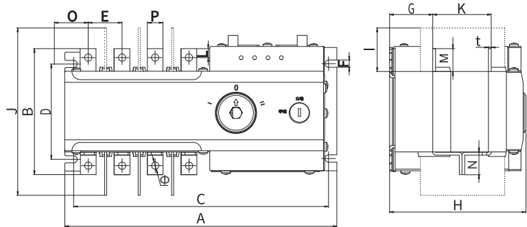
RDH5DS-160~630外形
