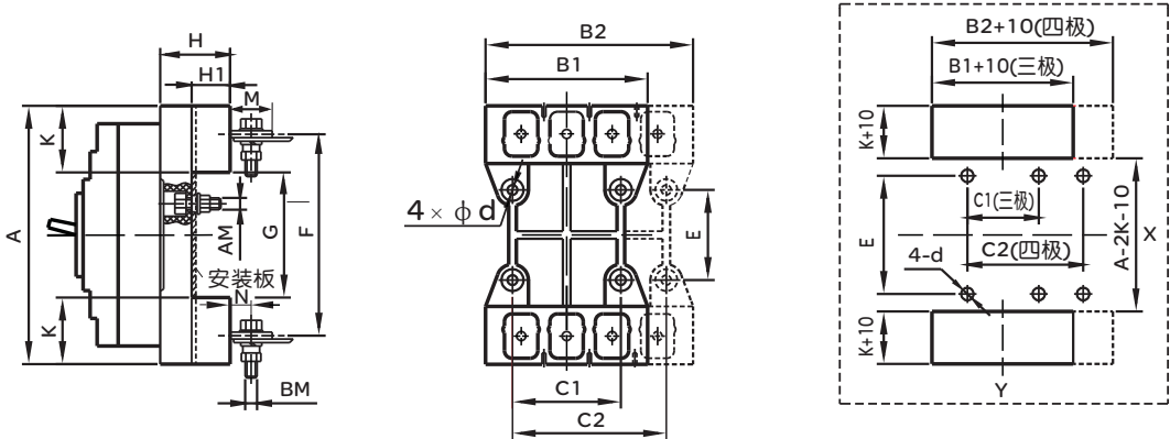
图9 RDM1系列插入式外形及安装板开孔尺寸图
