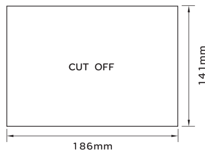
控制器开孔尺寸
