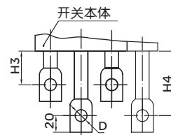
RDM1-400、630、800板后接线
