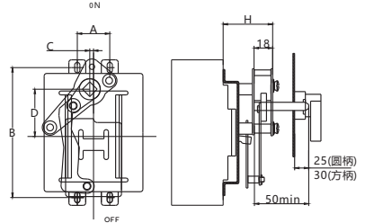
1250壳架SC2系列手操尺寸图
