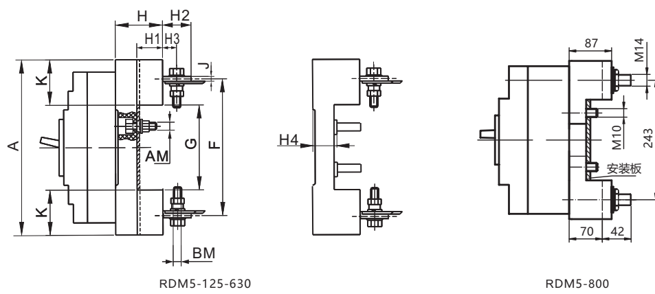
RDM5系列插入式板后外形尺寸及安装板开孔尺寸图
