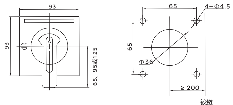
方形延伸旋转手柄开孔尺寸图
