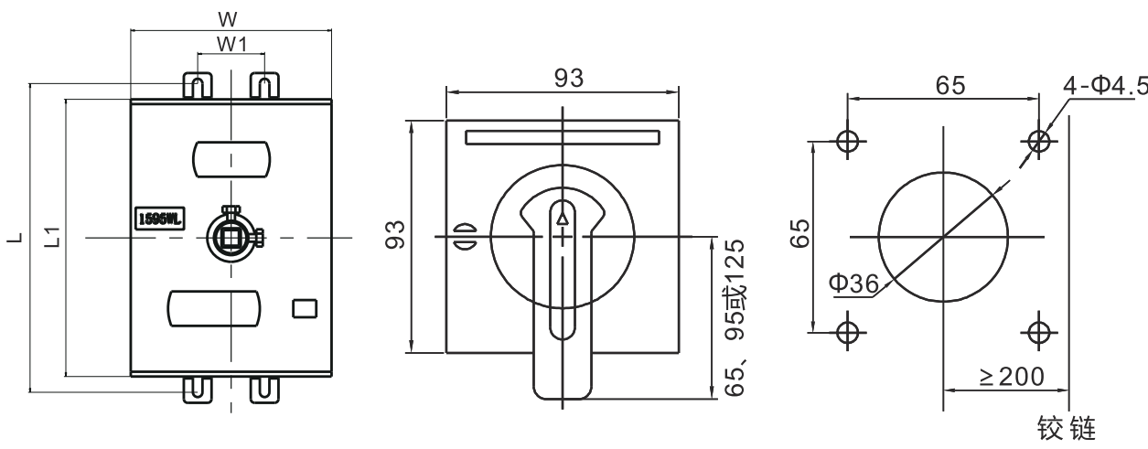
方形延伸旋转手柄开孔尺寸图
