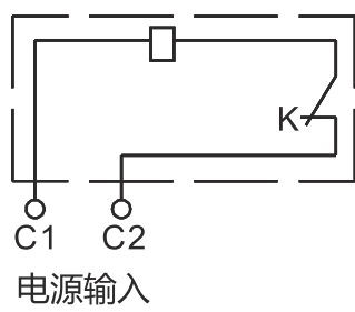
图1 AC 230V、400V;DC24V接线图
