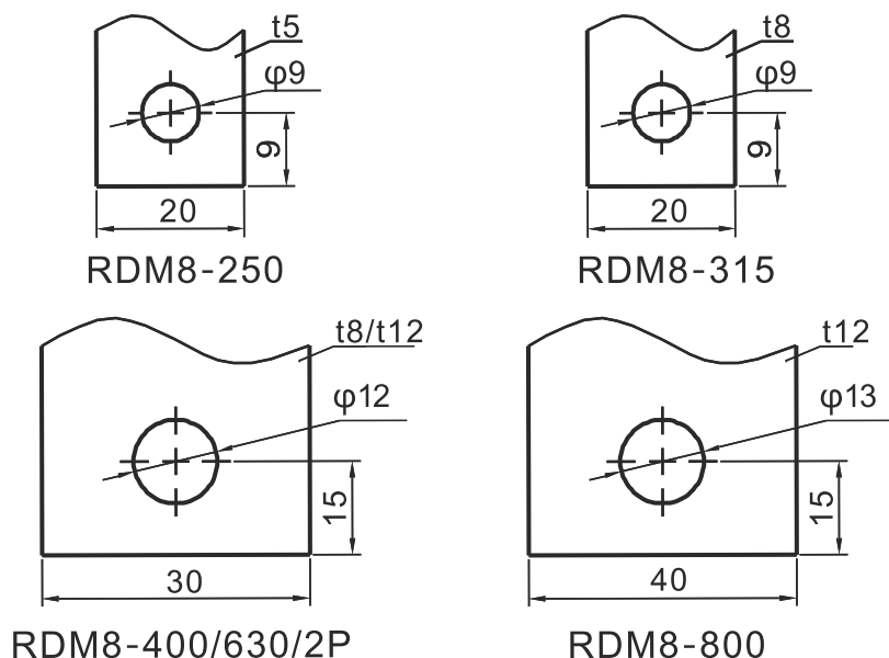
图2 RDM8系列推荐预制铜排尺寸
