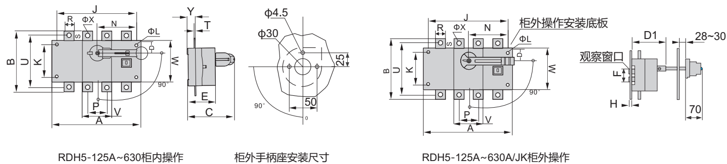
RDH5(HGL)-125A~630A负荷隔离开关外形及安装尺寸
