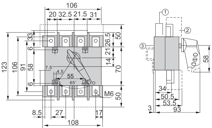
RDH5(HGL)-100 正面柜内操作
