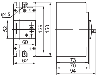
图4a RDM3L-125/2300
