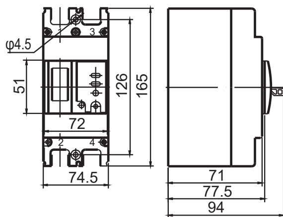
图4b RDM3L-250/2300
