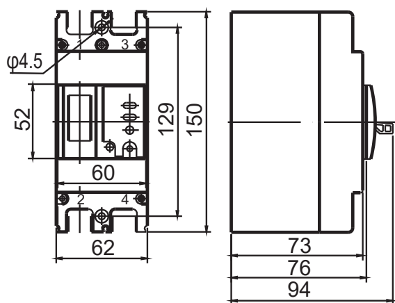
图4a RDM3L-125/2300
