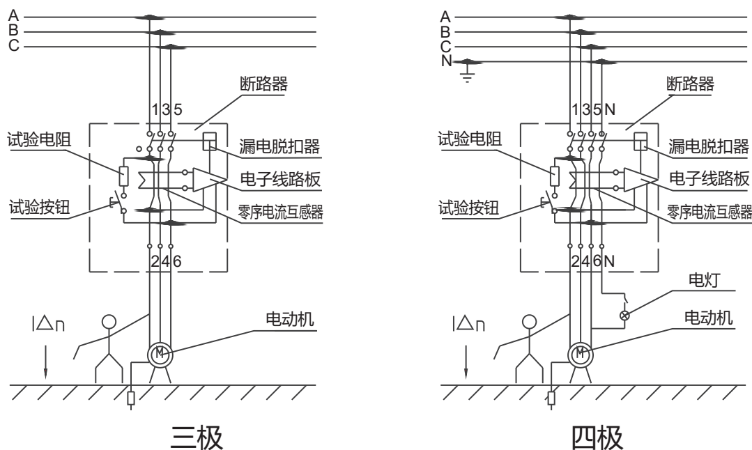
图1 工作原理
