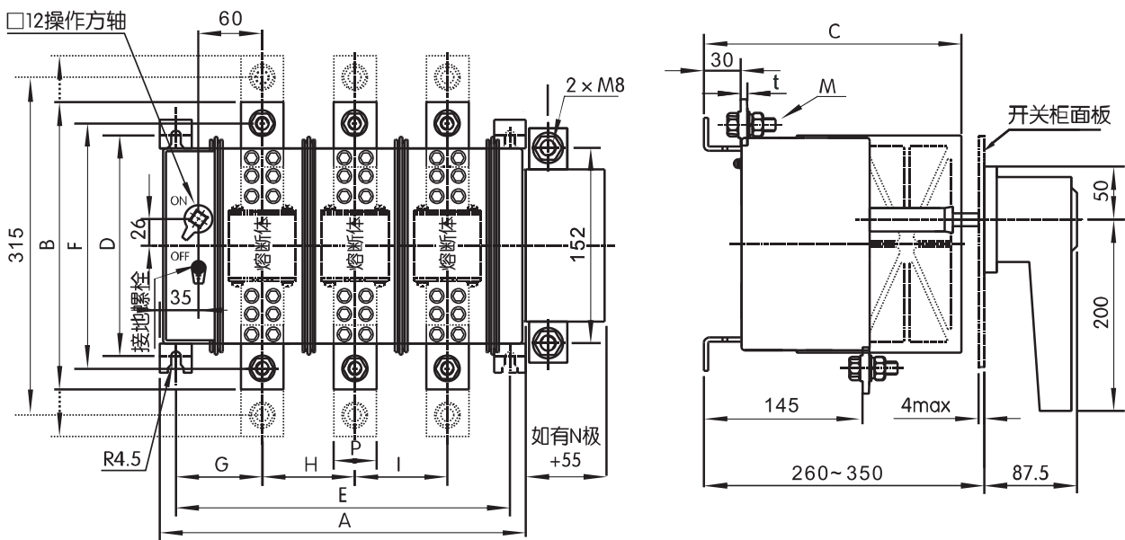
HH15(QSA)-630S、800S型外形及安装尺寸 800S型为双孔，为图样虚线部分
