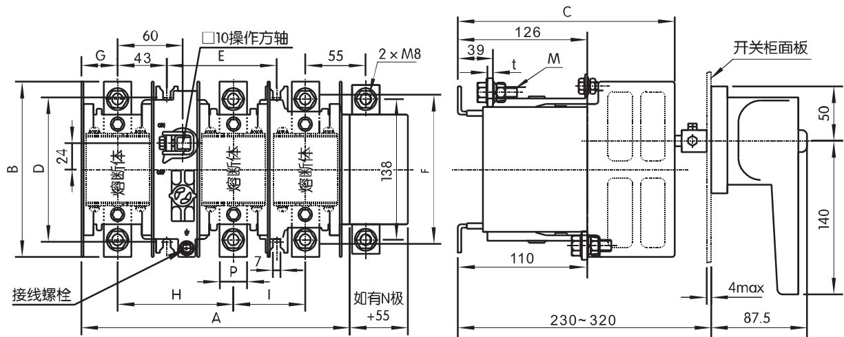
HH15(QSA)-250S、400S型外形及安装尺寸
