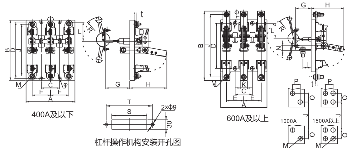
6.9 HS13中央杠杆操作机构刀开关外形及安装尺寸见图9、表10
