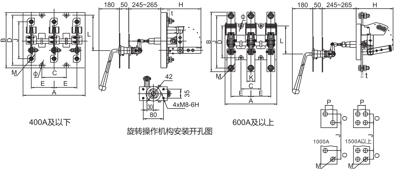
6.10 HD13BX中央旋转操作机构刀开关外形及安装尺寸见图10、表11
