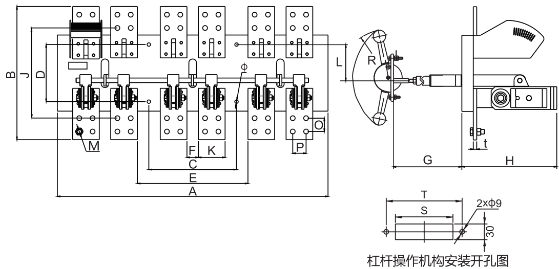
6.8 HD13 中央杠杆操作机构开启式刀开关外形及安装尺寸见图8、表9
