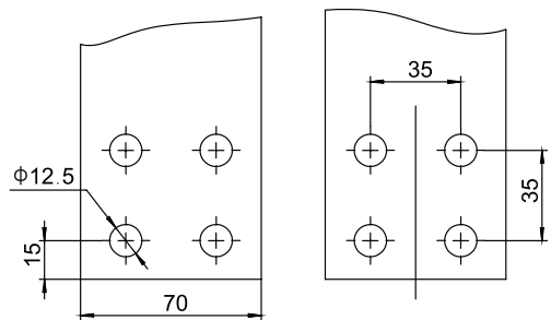
HD13-3000/31、41接线排示意图
