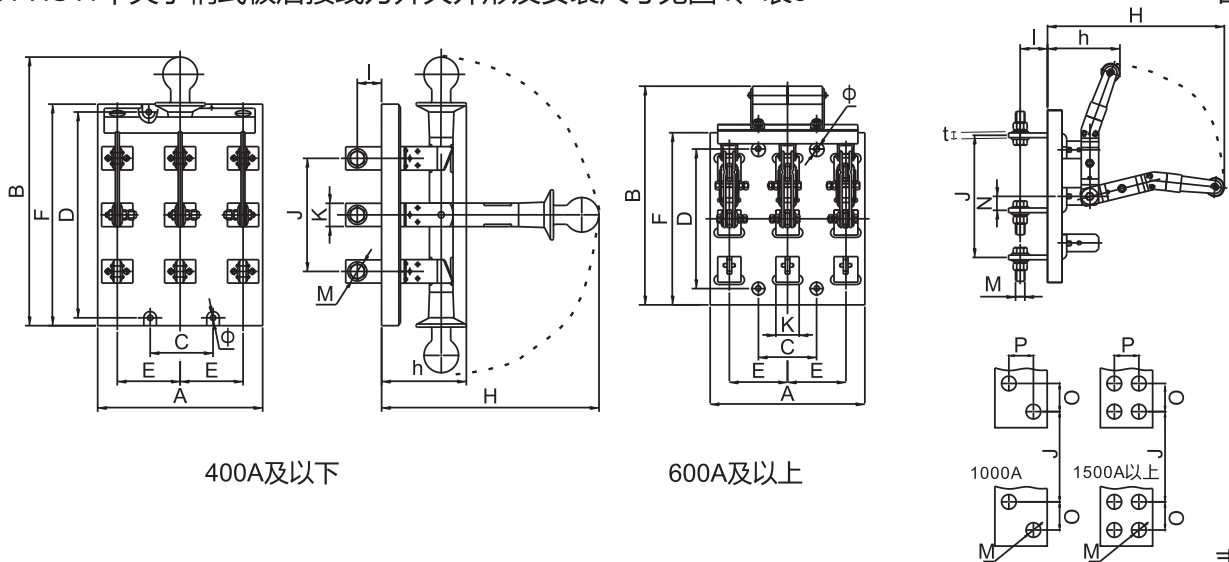
6.4 HS11中央手柄式板后接线刀开关外形及安装尺寸见图4、表5
