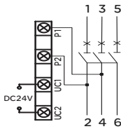
图2 DC24V接线图
