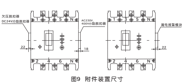
图9 附件装置尺寸
