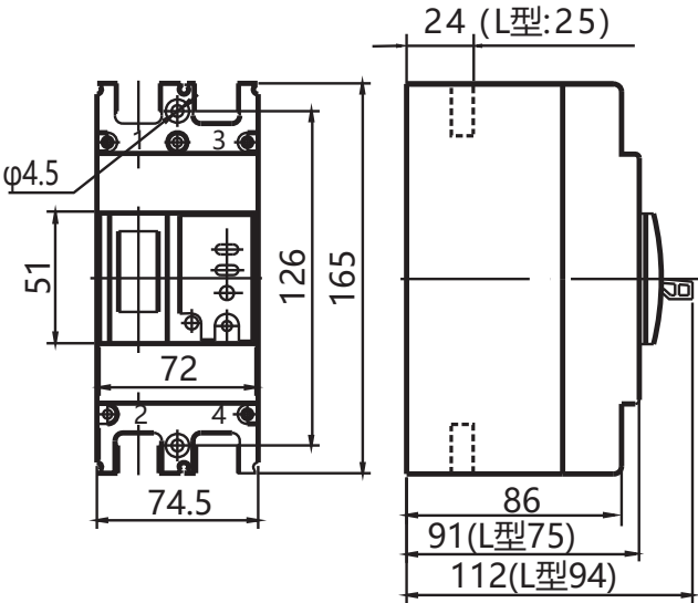
图8b RDM1L-250M/2300
