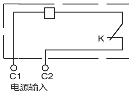
图3 AC50Hz、230V、400V接线图
