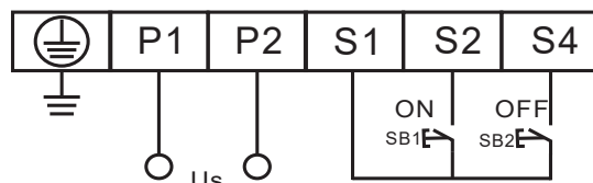
图5 CD2电动机接线图
