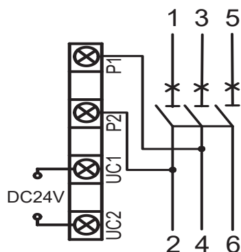
图2 DC24V接线图
