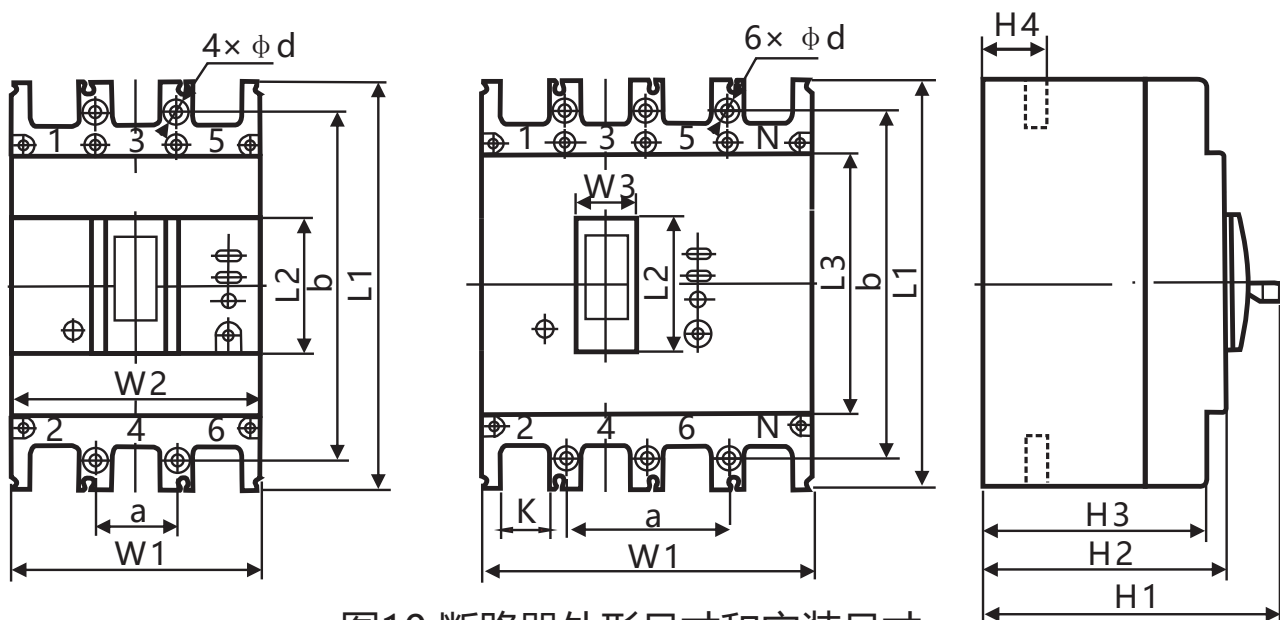
图10 断路器外形尺寸和安装尺寸 表10 断路器外形尺寸
