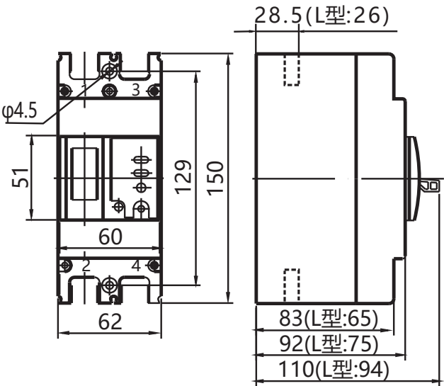
图8a RDM1L-125M/2300
