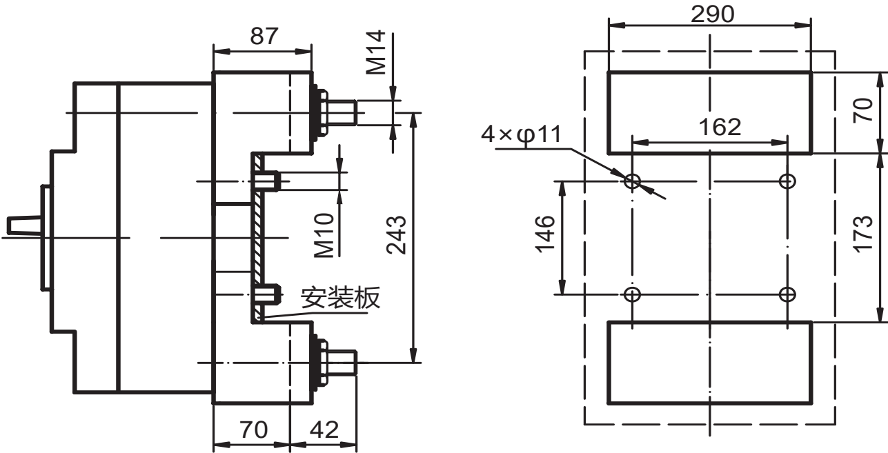
图14 RDM1L-800四极插入式板后外形及安装板开孔图
